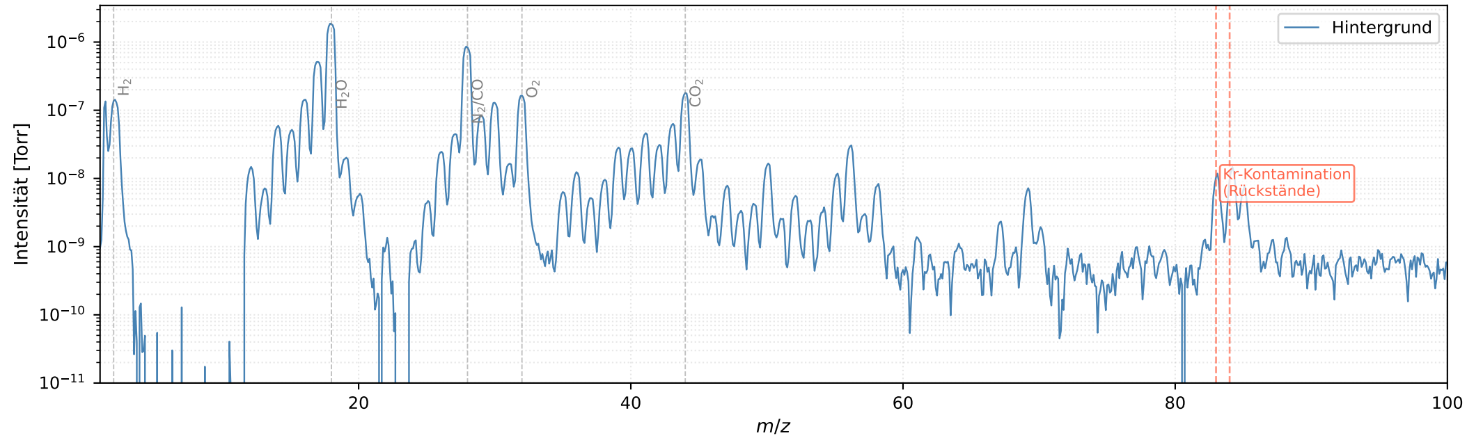
(a) Vollständiges Hintergrundspektrum (vor Kr-Einlass)
