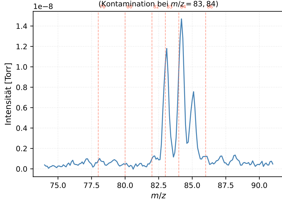
(b) Hintergrund im Kr-Bereich (Kontamination bei m/z = 83, 84 )
