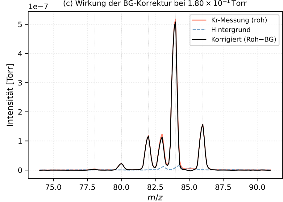
(c) Wirkung der BG-Korrektur bei 1.80 \times 10^{-1} Torr
